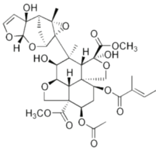
Azadirachtin
